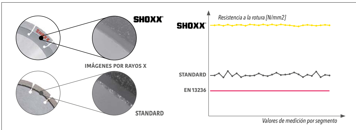
Soldado profundo y libre de poros de los segmentos SHOXX
